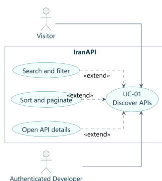
شکل ۲-۳ نمودار PlantUML مورد کاربرد UC-01
